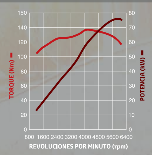
Datos con curva de potencia y torque.
